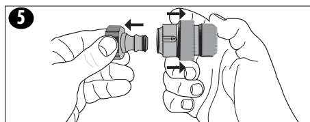
Figure 5 / 5A - Détacher les deux extrémités de l'adaptateur à raccordement rapide (M), tel qu'illustré à la figure 5, puis brancher l'extrémité fileté de la plus grande moitié (M2) au tuyau d'arrosage, tel qu'illustré à la figure 5A.
