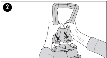
Figure 2 - Installer la poignée supérieure (N), tel qu'illustré.
